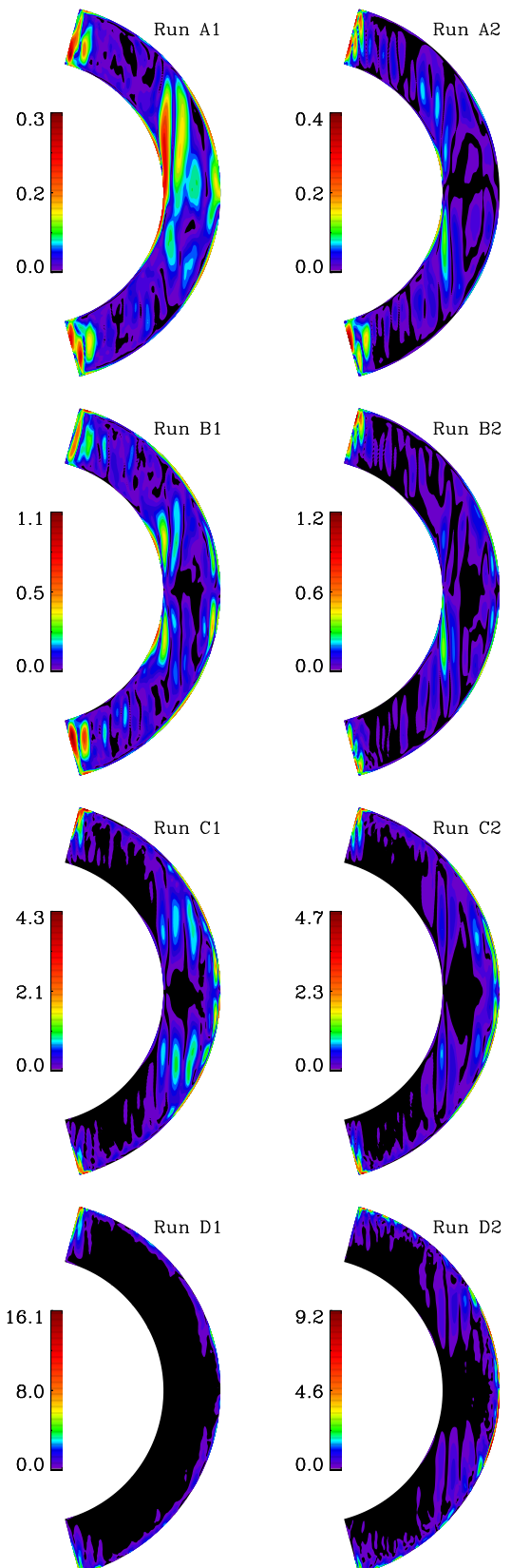
FIG. 13.— Local dynamo parameter c_U from Sets A, B, C, and D.
